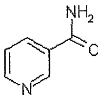
Nicotinamide (NA)
