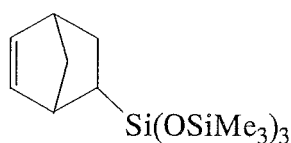
Monomer A
