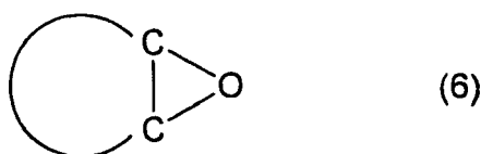
[Chem. 3]
