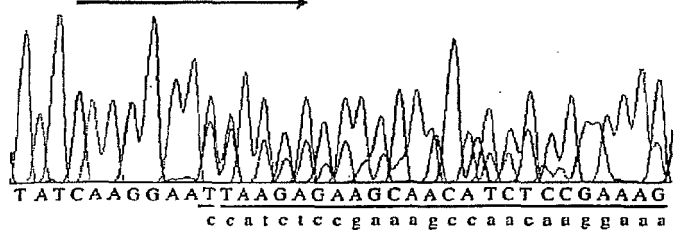
del L747-T751insS (antisense)
