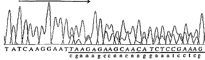
del L747-P753insS (antisense)
