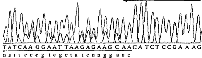
del L747-T751insS (antisense)
