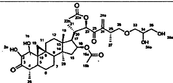
Verbindung 67
