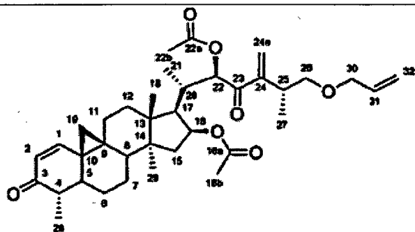
Verbindung 65
