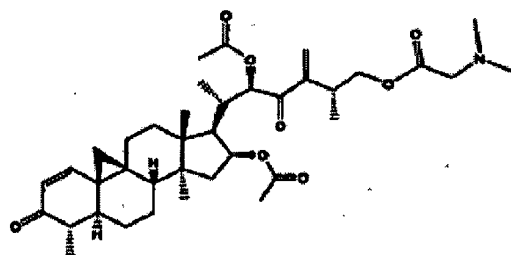
Verbindung 50
