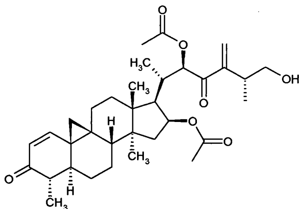
(neoboutomellerone).
