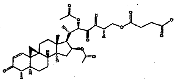
Verbindung 56
