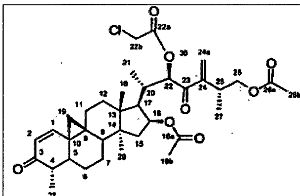
Verbindung 49
