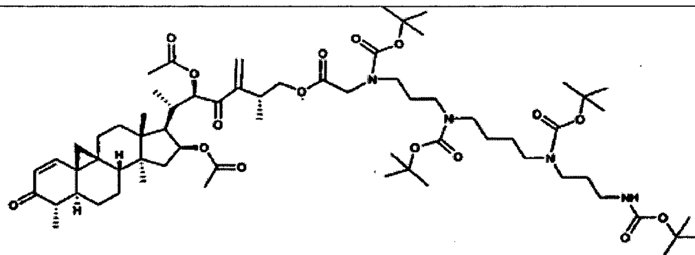
Verbindung 70
