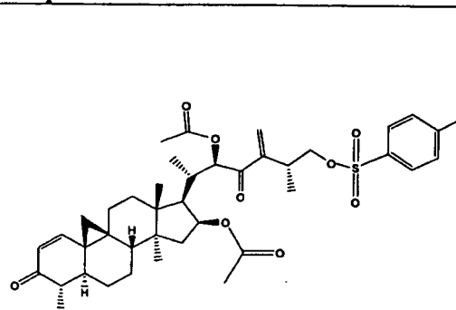
composé 38
