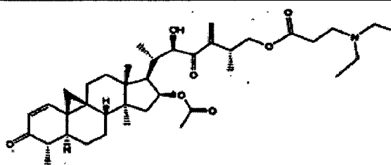
Verbindung 54
