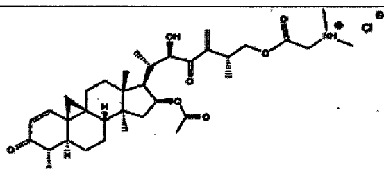
Verbindung 53
