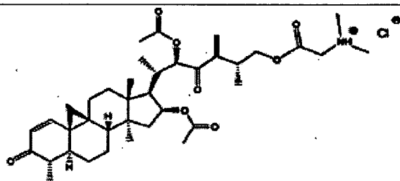
Verbindung 51
