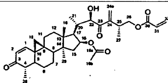
Verbindung 55
