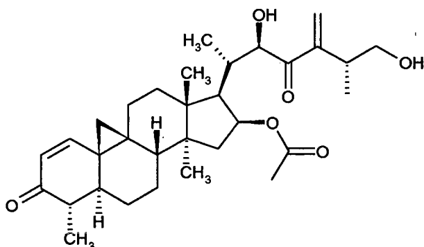
(22-déacétyl-neoboutomellerone)
