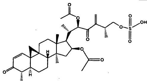
composé 35
