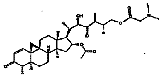
Verbindung 52
