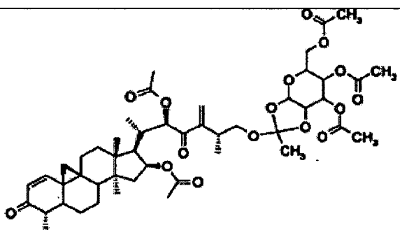
Verbindung 69
