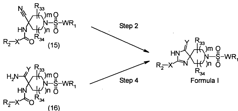
Scheme 5 (Method B)
