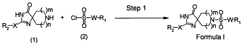
Scheme 1 (Method A)
