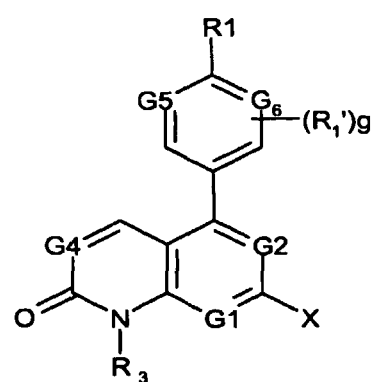
(Va)
