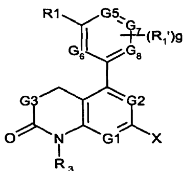
(VIh) or
