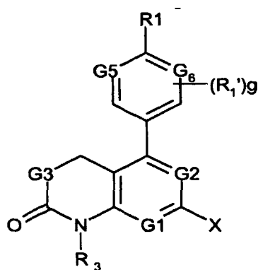
(V)
