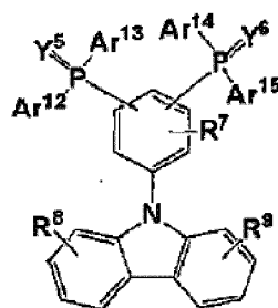
[Formule chimique 4]
