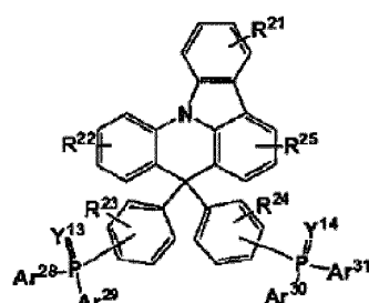
[Formule chimique 8]
