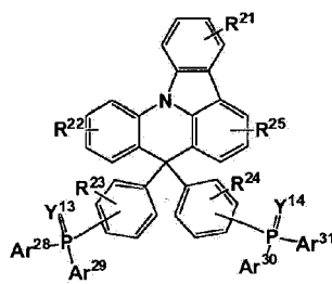
[Chemische Formel 8]
