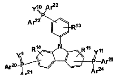
[Formule chimique 6]
