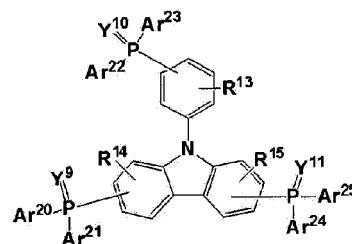
[Chemische Formel 6]
