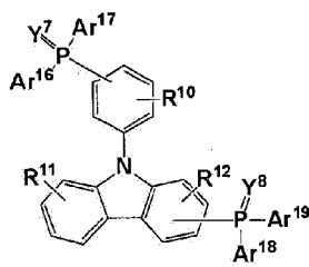
[Chemische Formel 5]
