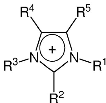
Imidazolium
