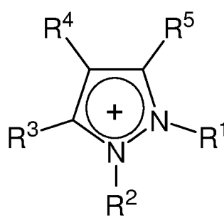
Pyrazolium
