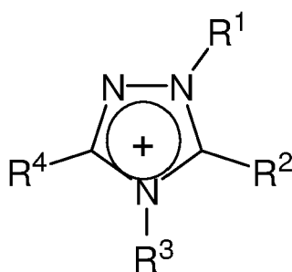
Triazolium
