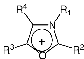
Oxazolium
