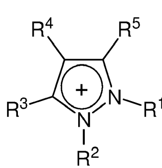
Pyrazolium
