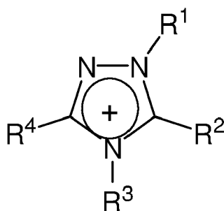
Triazolium
