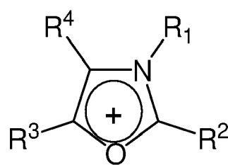
Oxazolium
