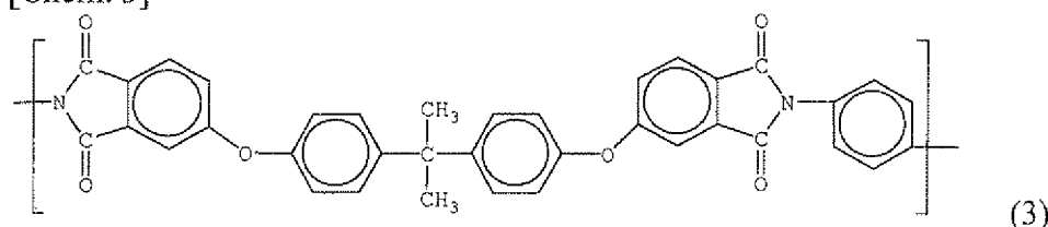
[Chem. 3]
