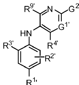
Formula (I-b)
