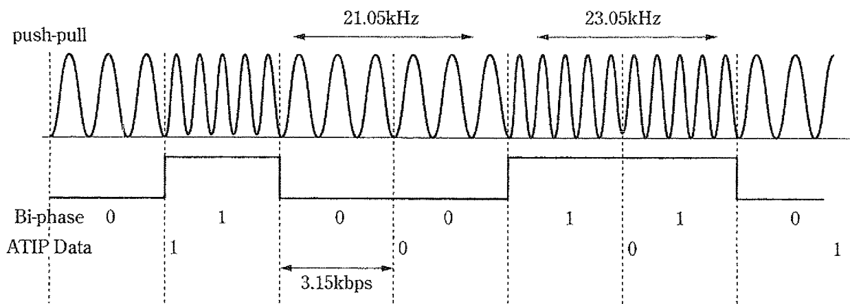
ATIP Encoding
