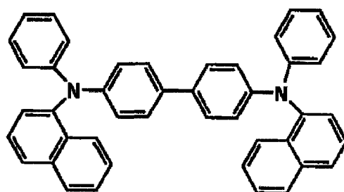
\alpha -NPD
