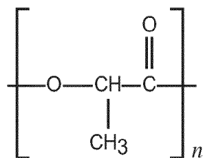
Poly(lactide)
