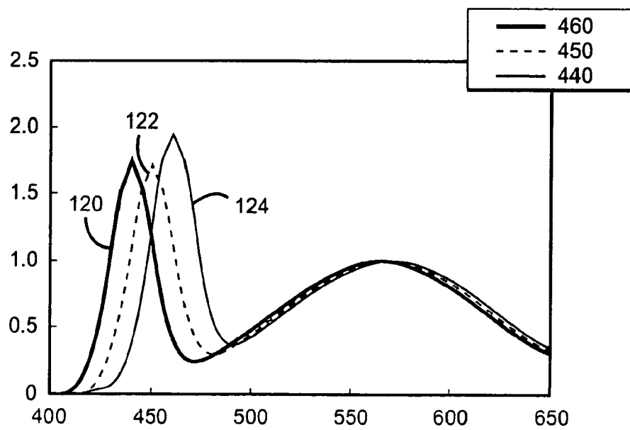
FIG. 4f
