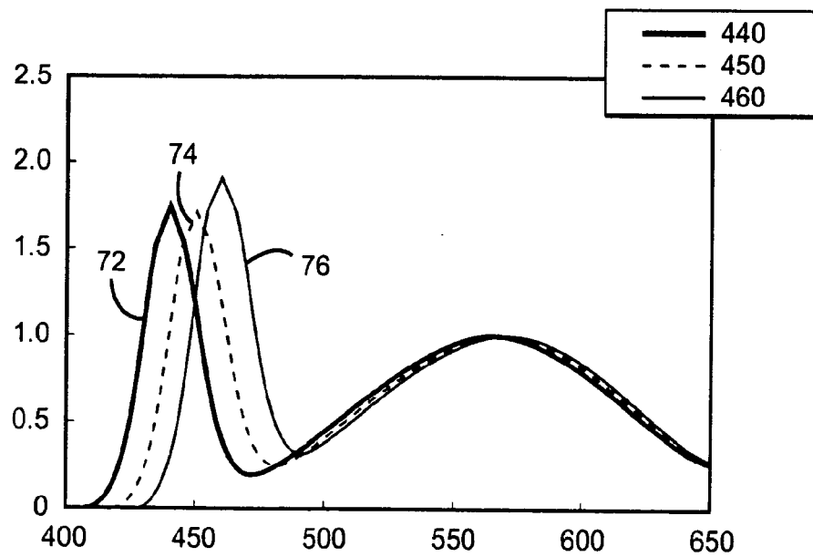
FIG. 3g
