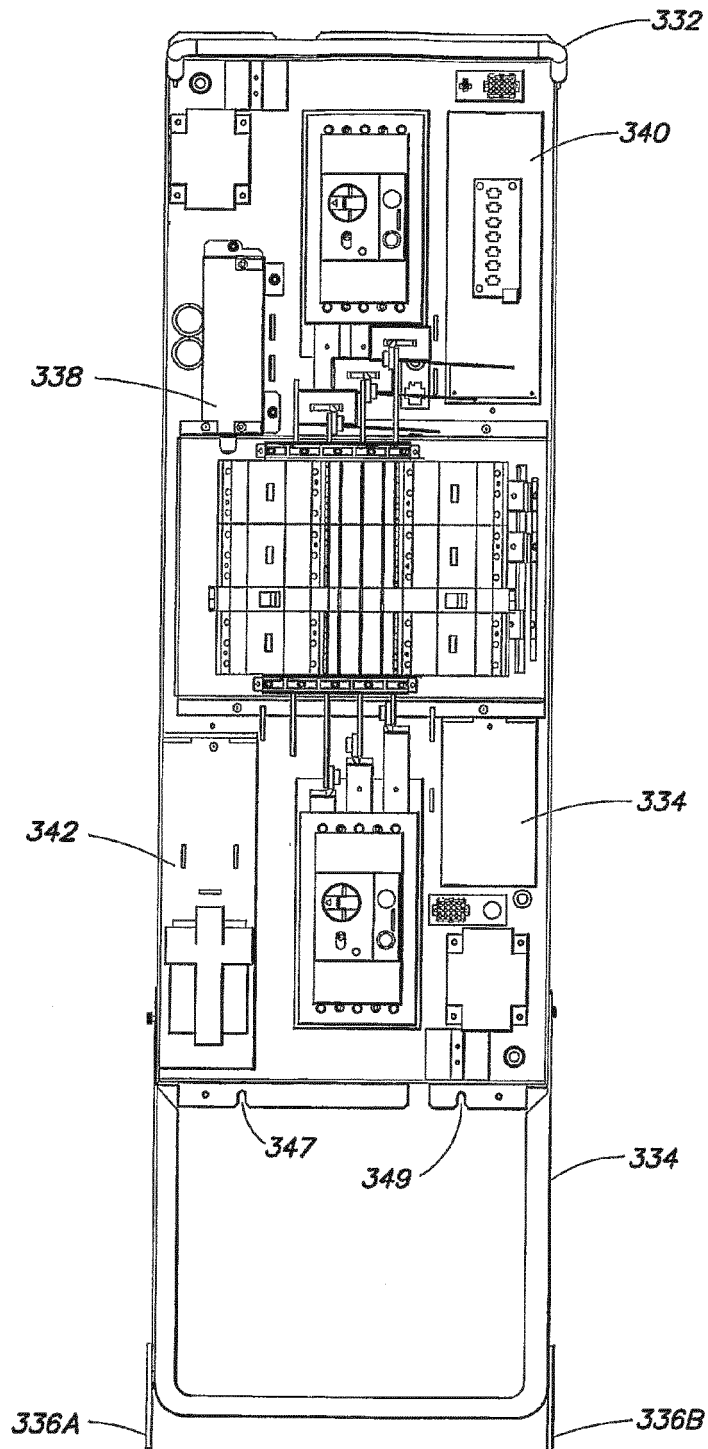
FIG. 9B
