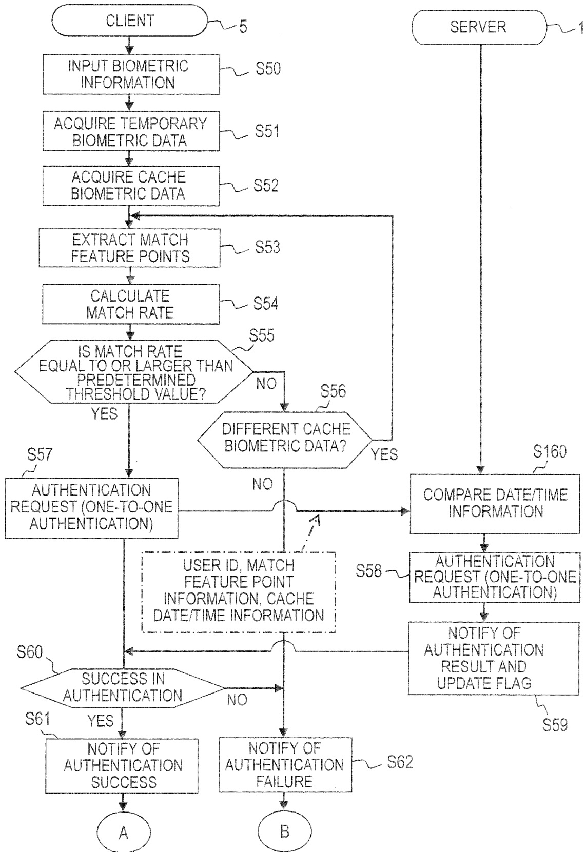
FIG. 16A
