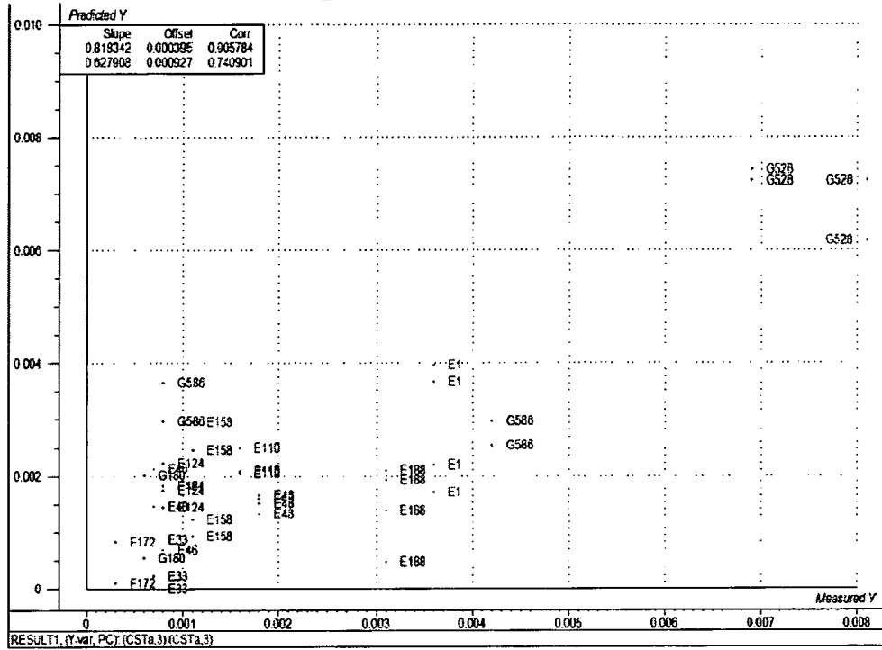
FFT vs OTR - 29 data points
