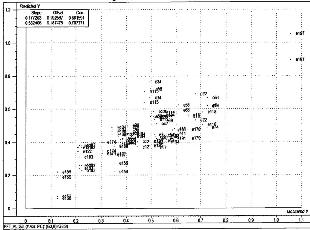
FFT vs OTR - 49 data points
