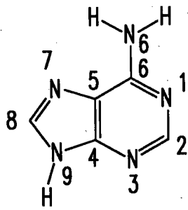
Adenine (Ade)
