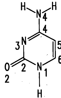
Cytosine (Cyt)
