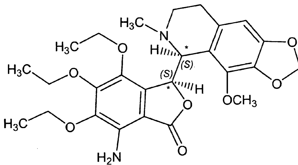
Isomer D2
