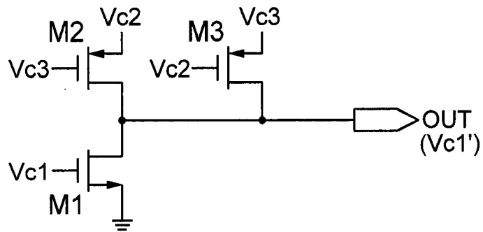
【FIG. 6B】 113-2
