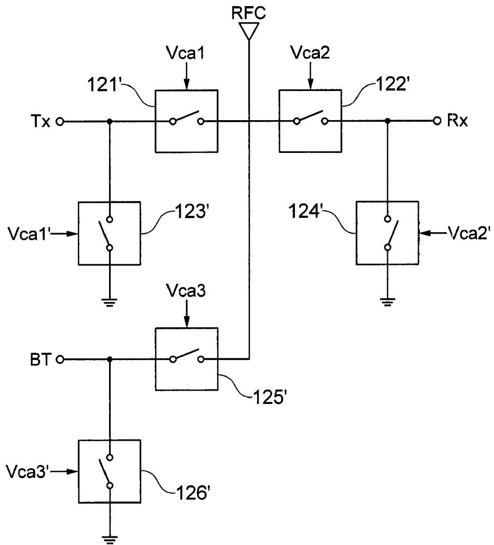
【FIG. 5】 120'
