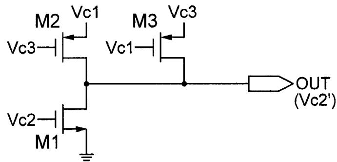
【FIG. 6C】 113-3
