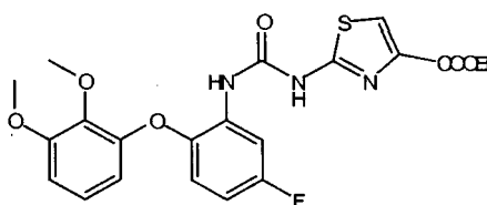
Novo Nordisk IV
