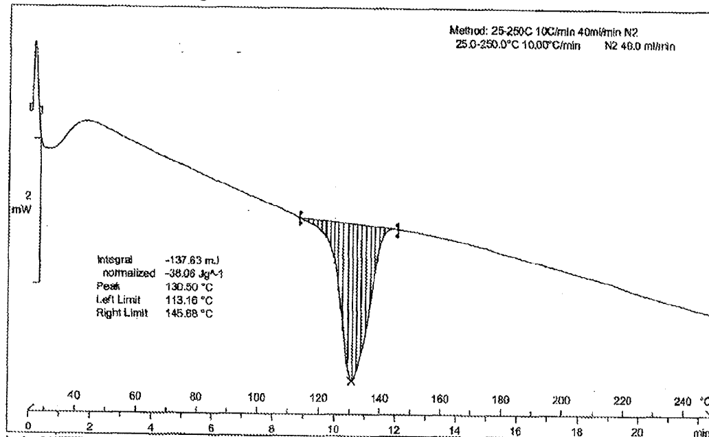
Figure 87: DSC thermogram of Dasatinib form AV
