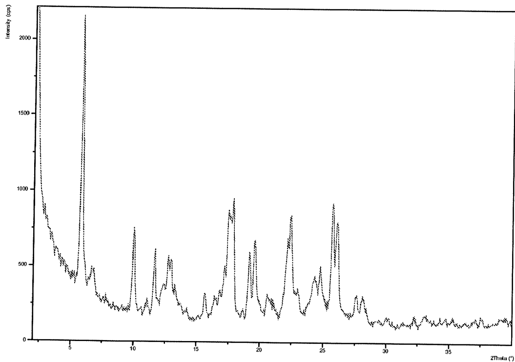
Figure 45: PXRD pattern of Dasatinib form AV
