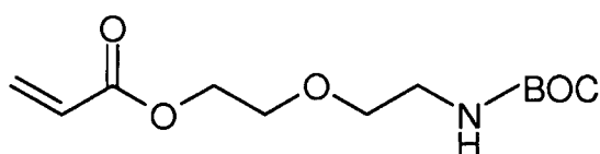
BAEEA
