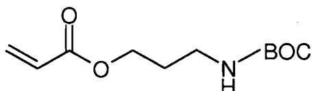
BAPA
