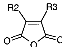
maleic anhydride
