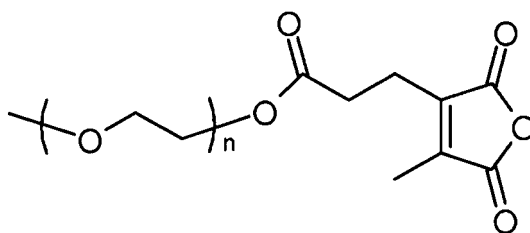
CDM-PEG
