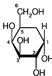
galactose
