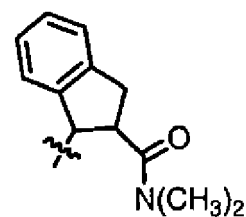
(VII)-ix
