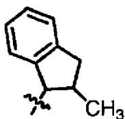
(VII)-ii
