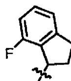
(VII)-xiii
