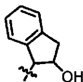
(VII)-xvi
