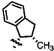
(VII)-xix
