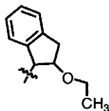
(VII)-xv
