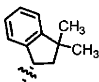
(VII)-xviii
