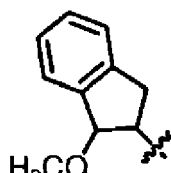
(VII)-vii
