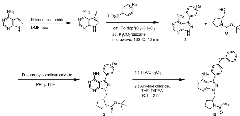
Scheme I.
