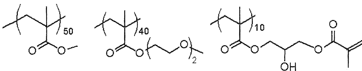
10 Binder polymer (1)
