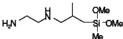
and N-(2-aminoethyl)-3-aminoisobutylmethyldimethoxysilane
