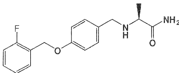
Ralfinamid (Ia)
