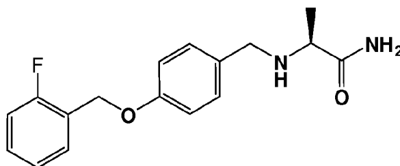
ralfinamide (1a)
