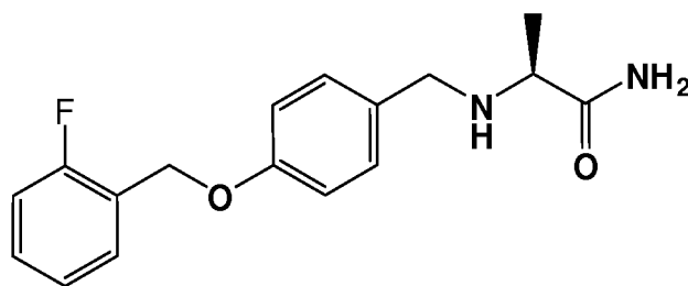
ralfinamide ( 1a )
