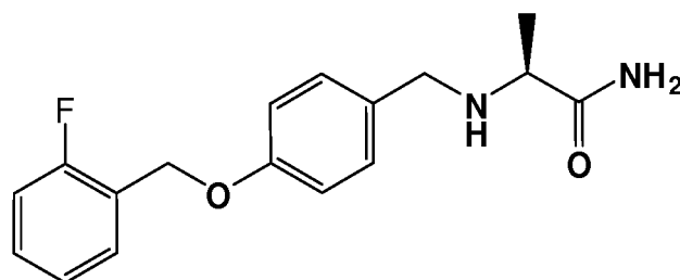
ralfinamide ( 1a )
