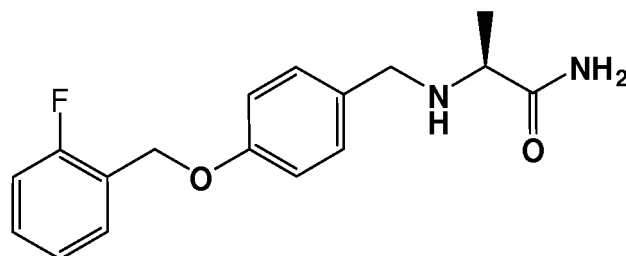
ralfinamide (1a)
