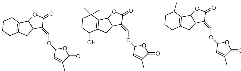
(II-22f)
