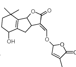
(II-22g)
