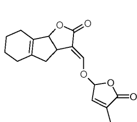
(II-22f)
