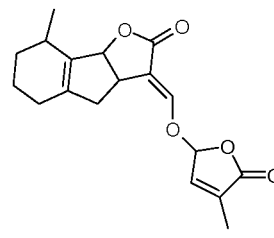
(II-22h)
