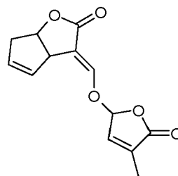
(II-22b)
