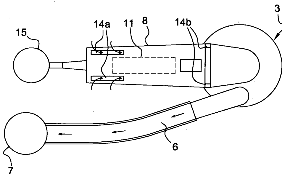
Fig. 4 Art antérieur
