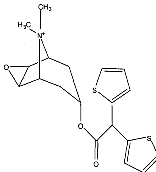
Tiotropium
