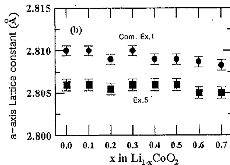
FIG.17B
