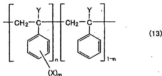
[Chem. 5]
