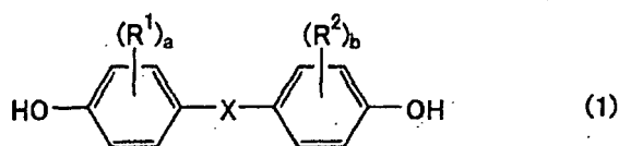
[Chem. 3]
