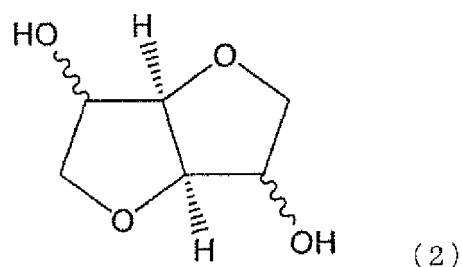
[Chem. 3]
