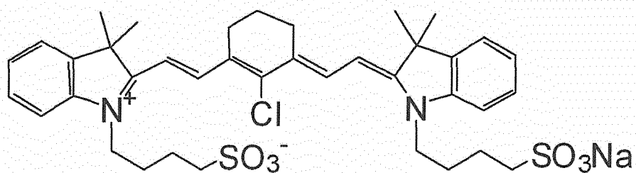
(I-iv) IR783
