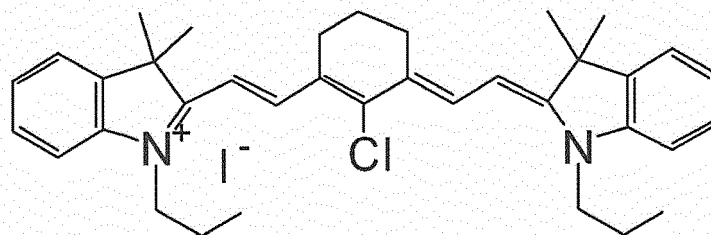
(I-viii) IR780
