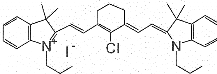
(I-viii) IR780
