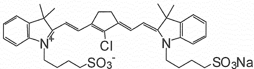
(I-v) IR806
