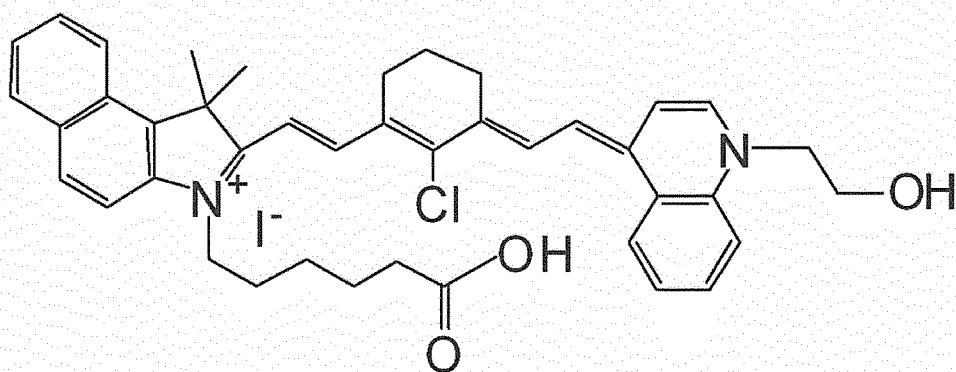
(I-vi) IC7-2
