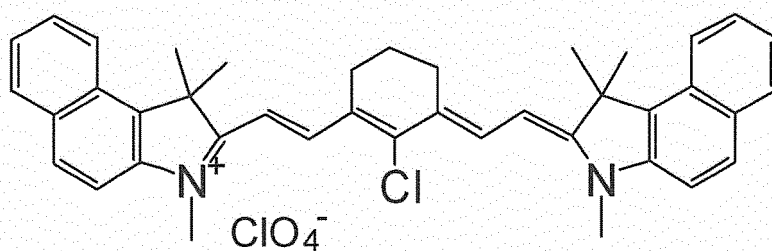
(I-xi) IR813
