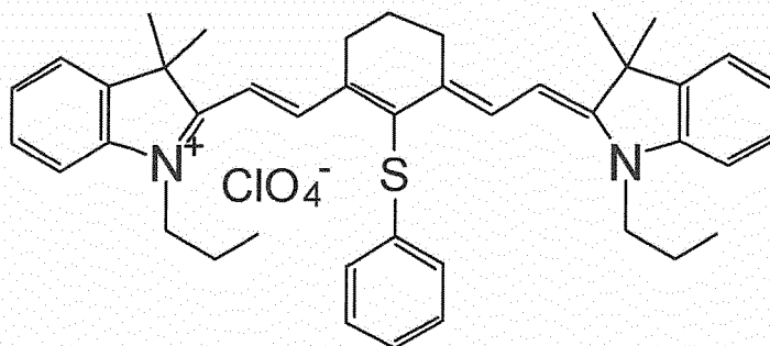
(I-ix) IR792
