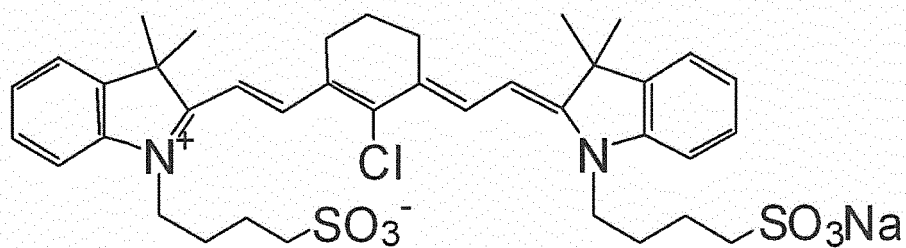
(I-iv) IR783
