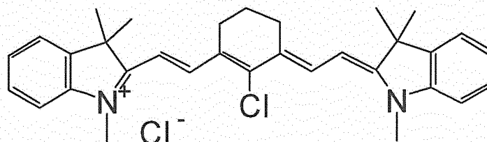
(I-vii) IR775
