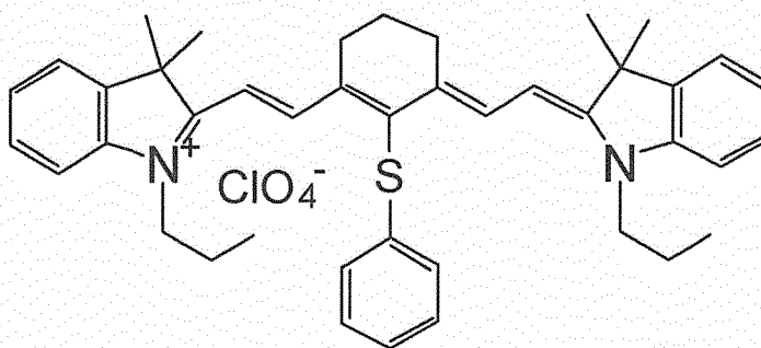
(I-ix) IR792
