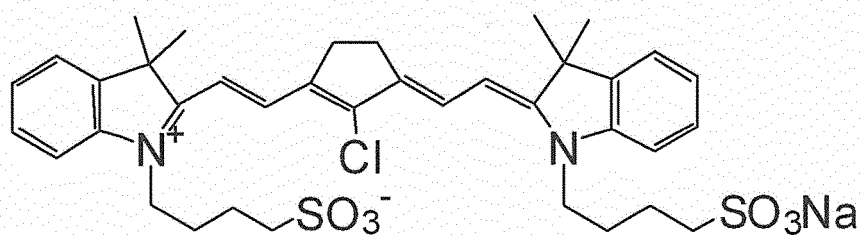
(I-v) IR806
