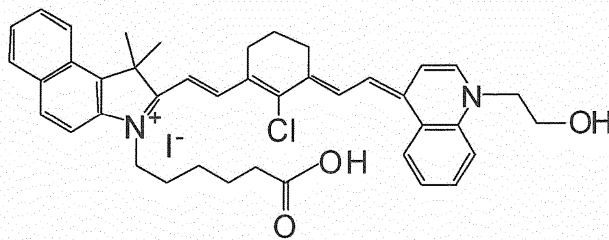
(I-vi) IC7-2
