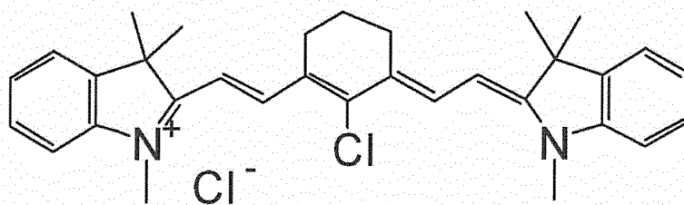
(I-vii) IR775
