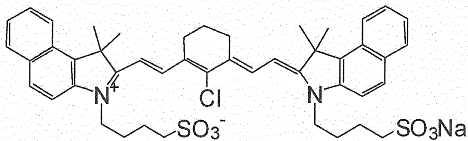
(I-iii) IR820
