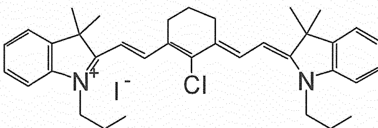
(I-viii) IR780
