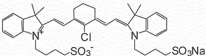
(I-iv) IR783
