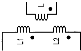
balun 980 FIG. 103
