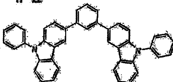
H-22
