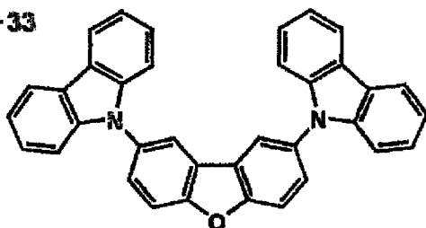
H-35
