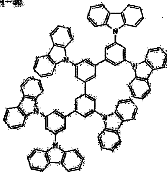
H-30
