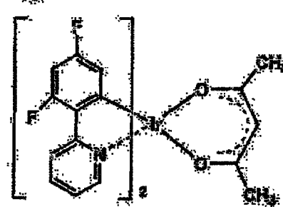
Ir-10
