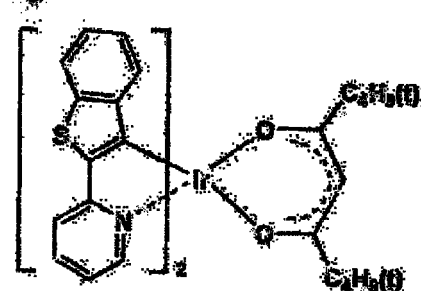
Ir-6
