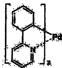
Pd-1
