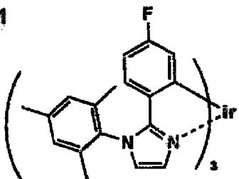
1-81
