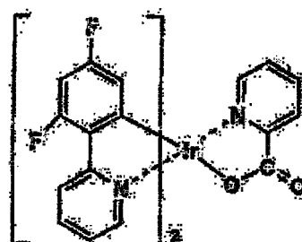
Ir-12
