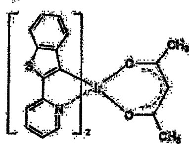
Ir-9
