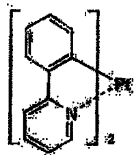
Pt-1
