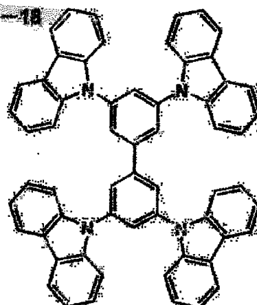
H-20
