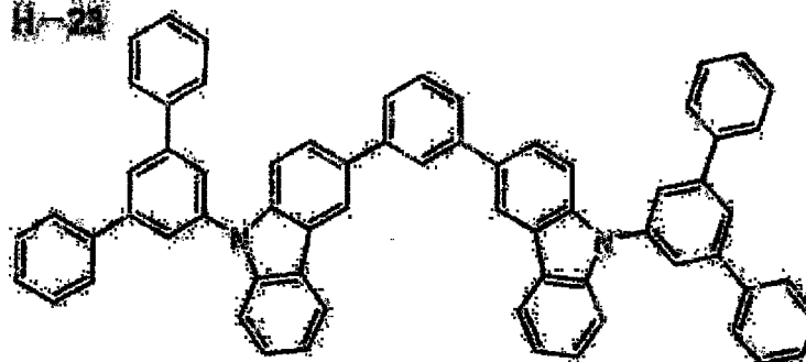
H-25
