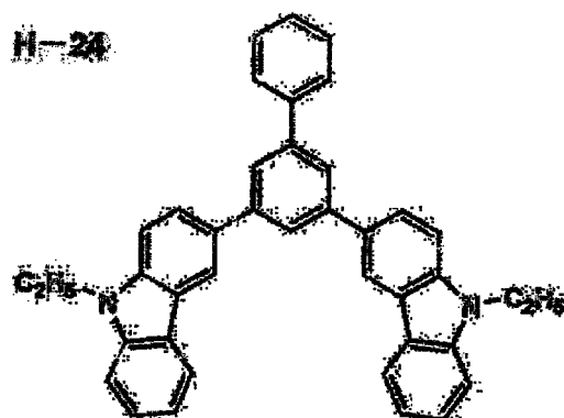
H-25
