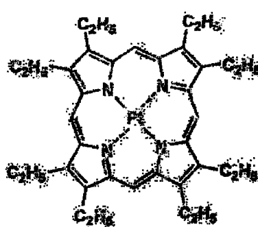
Pt-3
