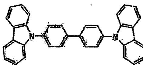
CBP
