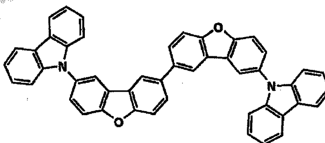
H-36
