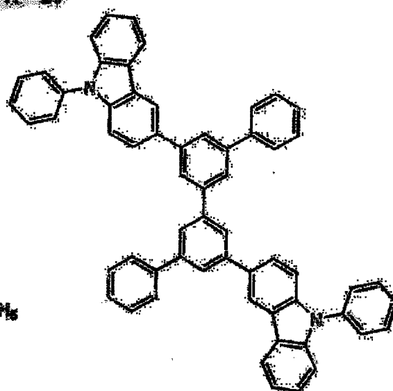
H-29
