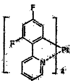
Pt-2
