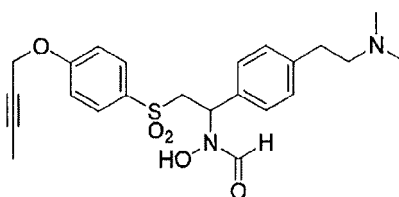
(I-20)
