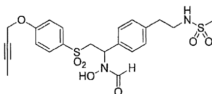
(I-22)
