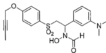
(I-9)
