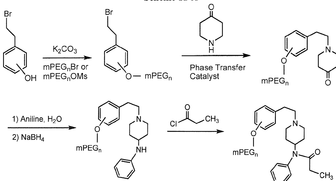
Scheme 11-A
