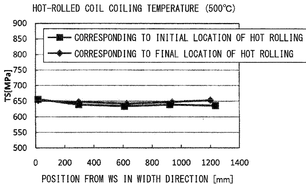
FIG. 3C
