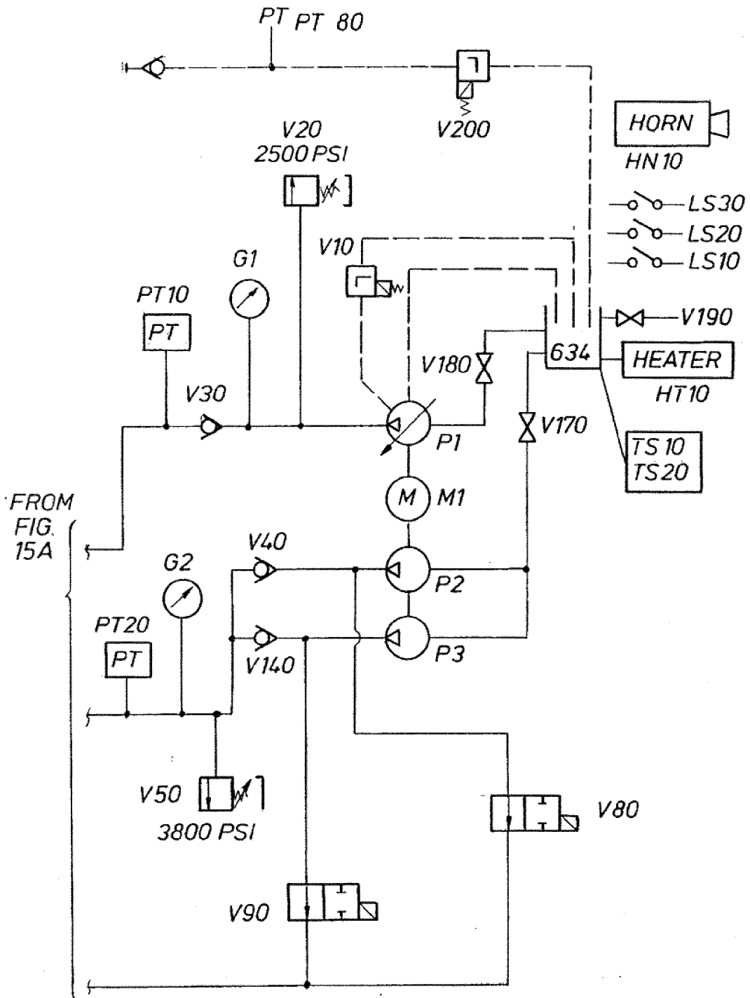
FIG.15B
