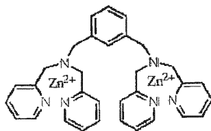
Zn 2+ -dipicolylamine
