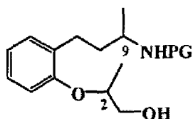
T101a [(2R,9R)-isomer] T101b [(2S,9S)-isomer] T101c [(2R,9S)-isomer] T101d [(2S,9R)-isomer]
