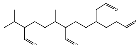
(a8)
