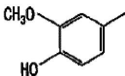
(VIII)
