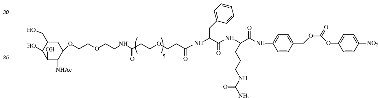
NAG-PEG7-Phe-Cit-PABC-PNP
