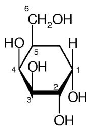
galactose
