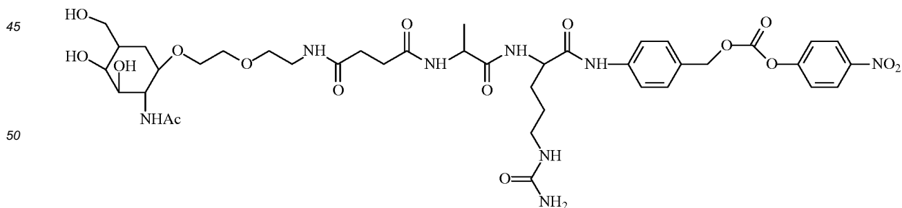
NAG-Ala-Cit-PABC-PNP
