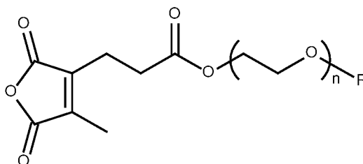
CDM-PEG
