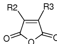
maleic anhydride
