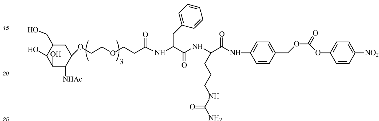
NAG-PEG4-Phe-Cit-PABC-PNP
