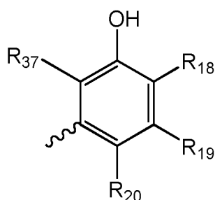
(IVa)
