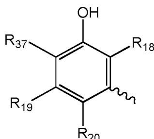
(IVb)
