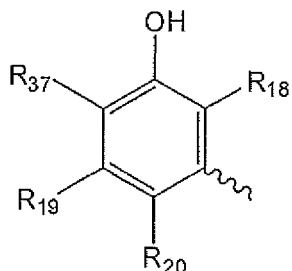
(IVb)
