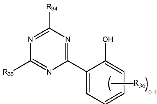
(VII)
