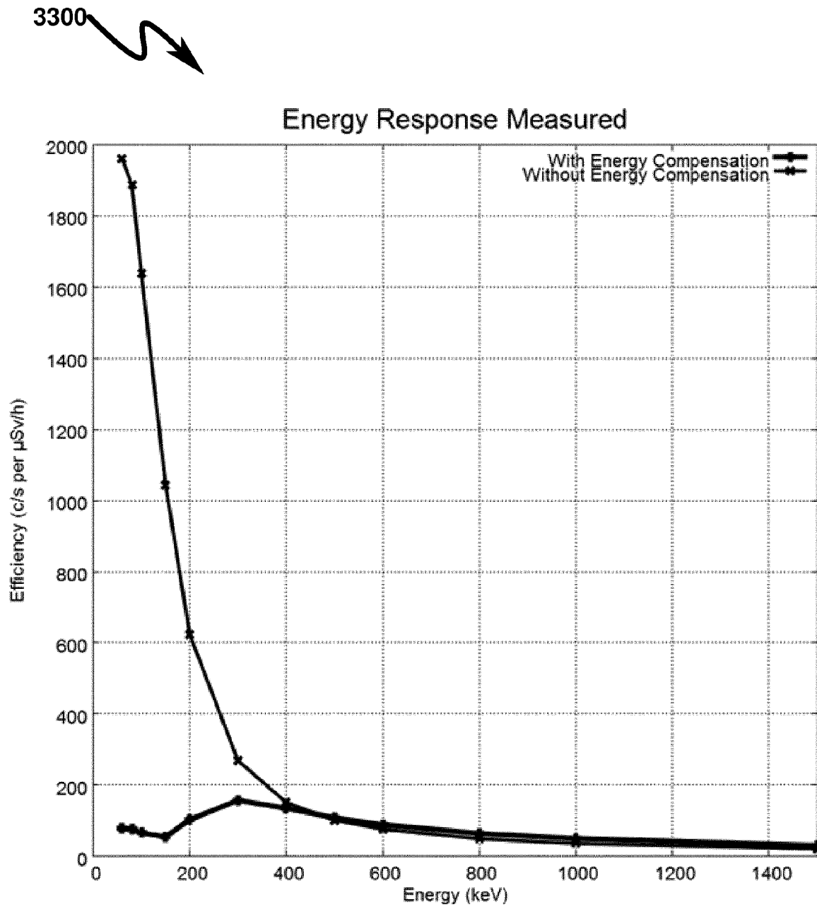
FIG. 33
