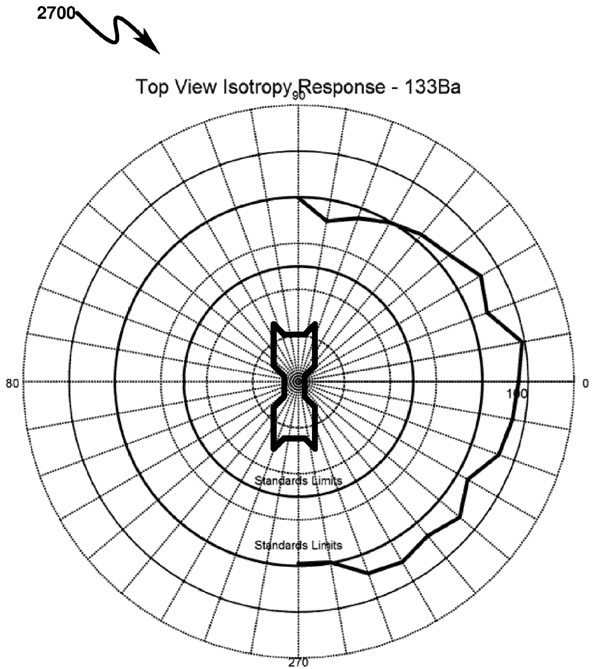
FIG. 27
