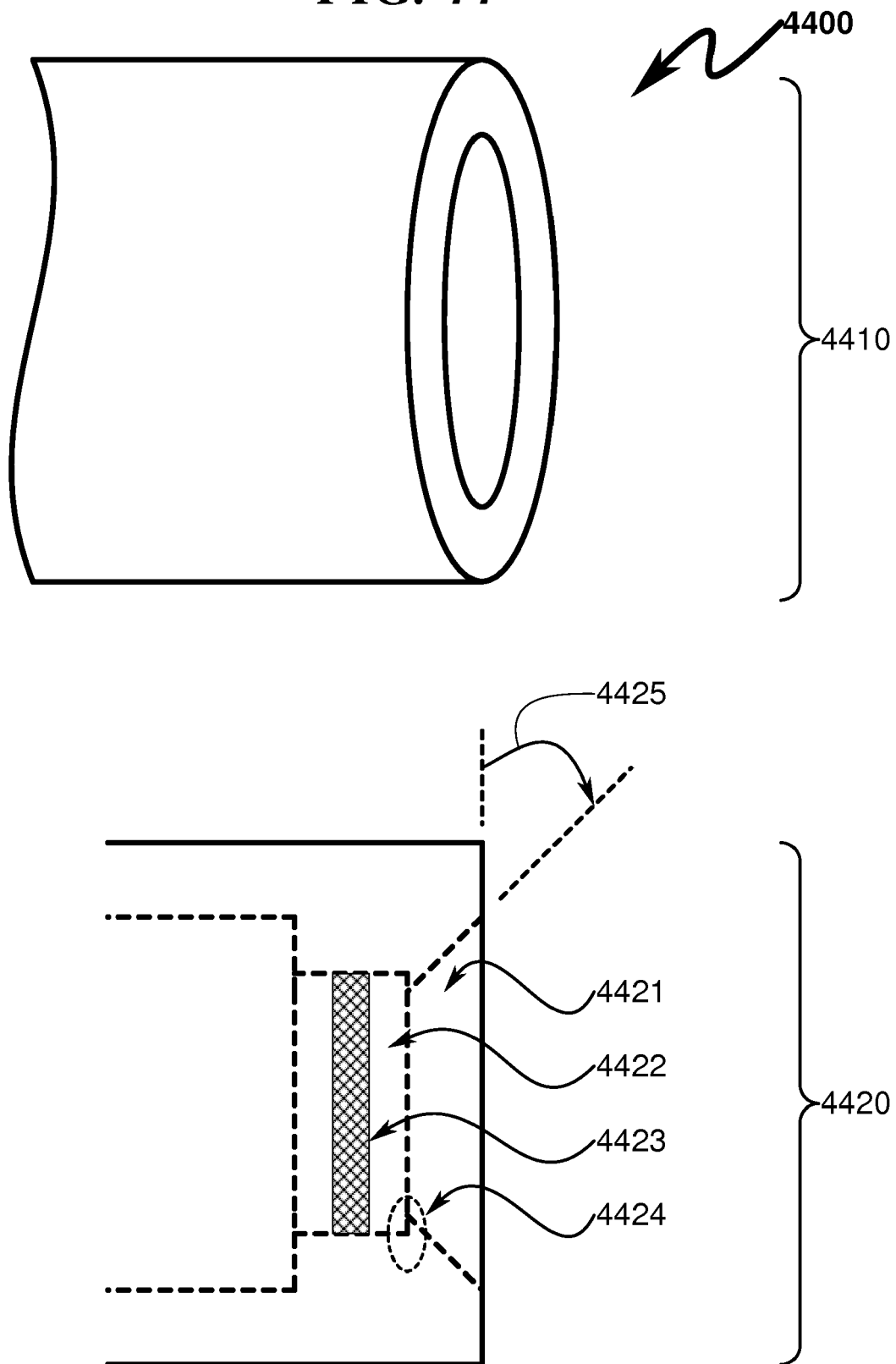
FIG. 44
