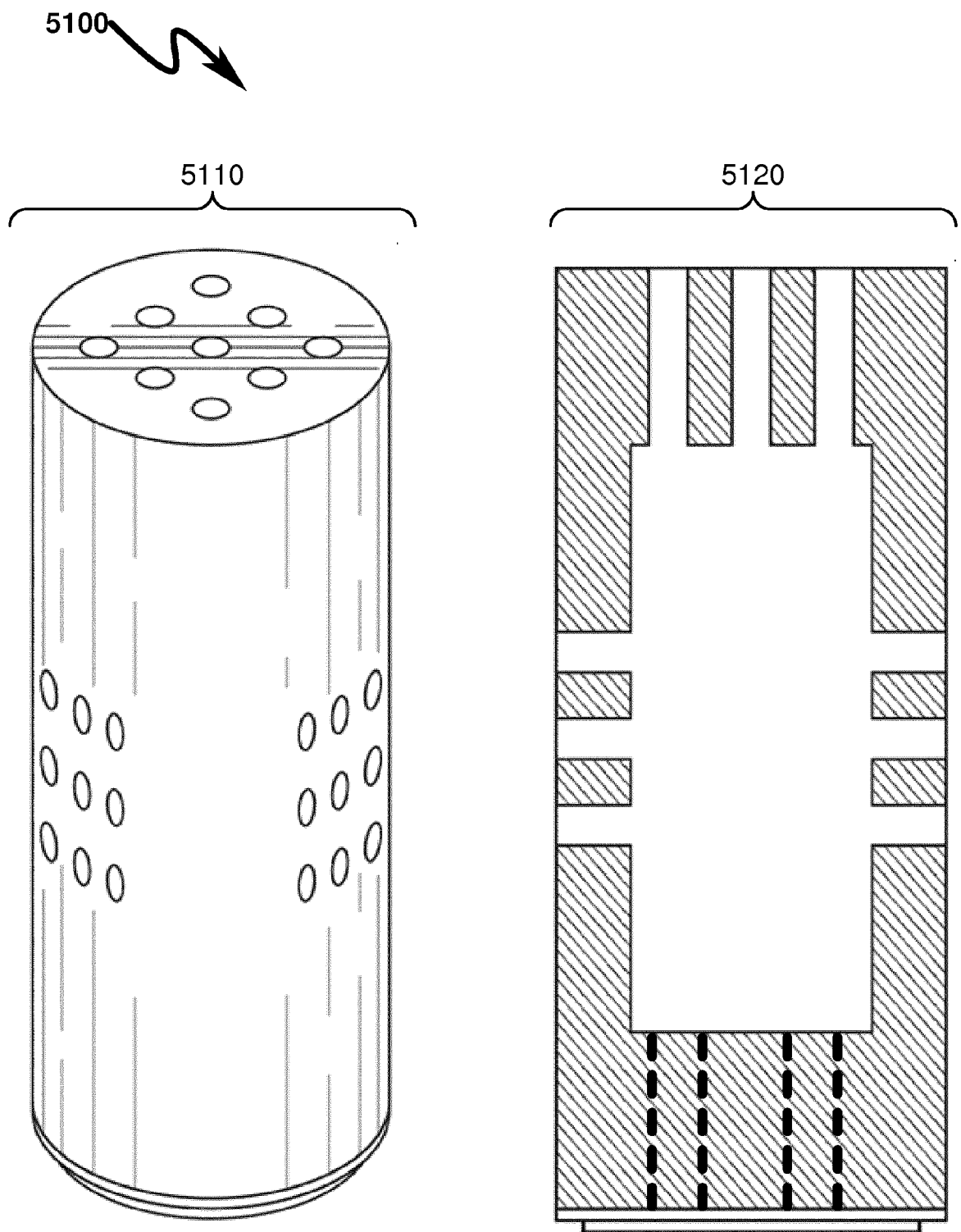
FIG. 51
