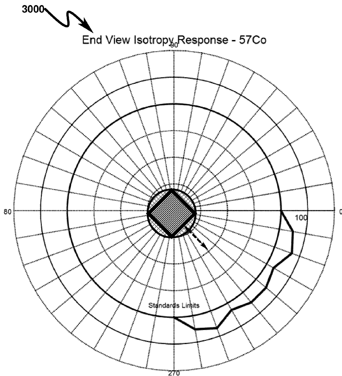
FIG. 30
