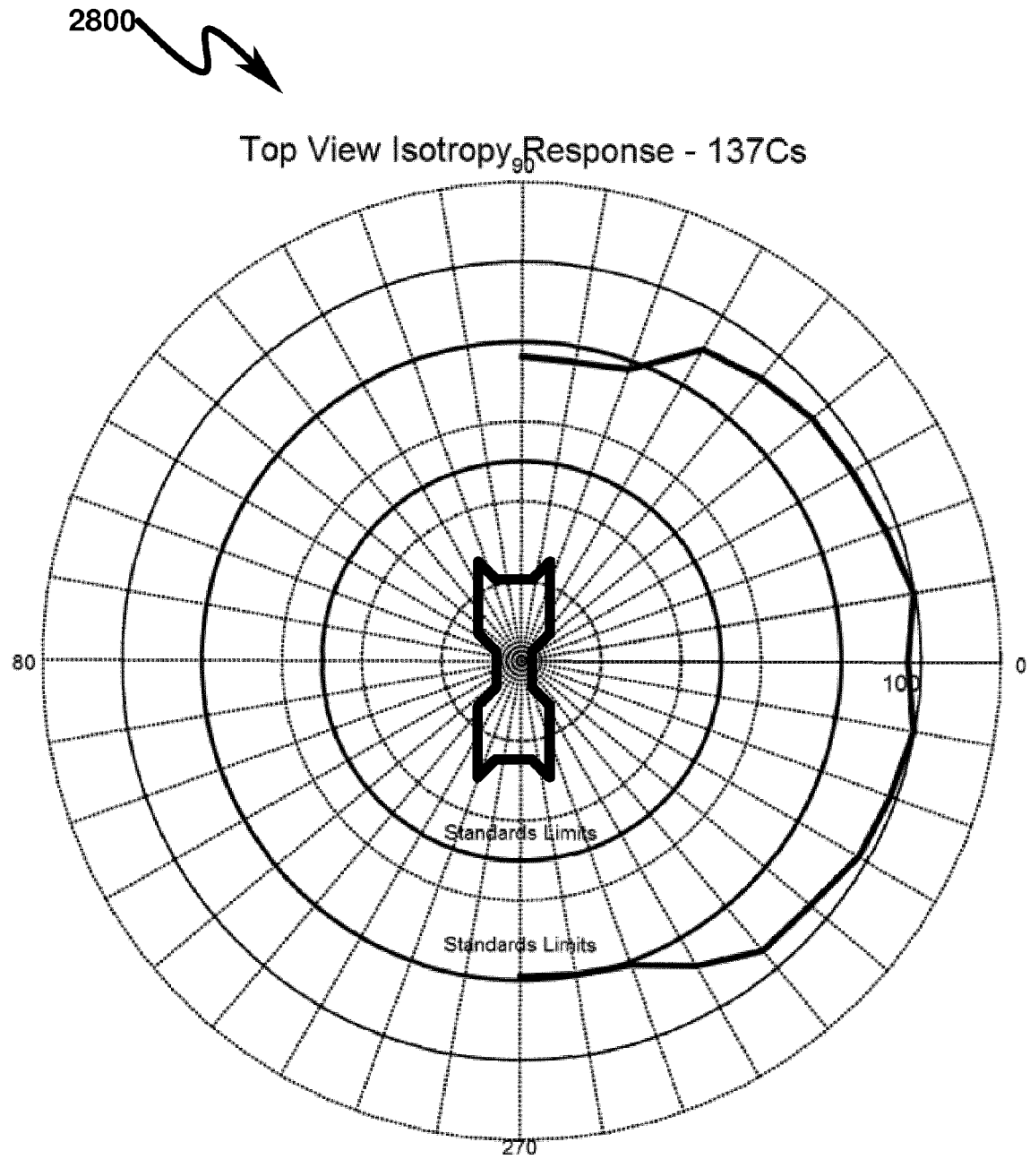
FIG. 28
