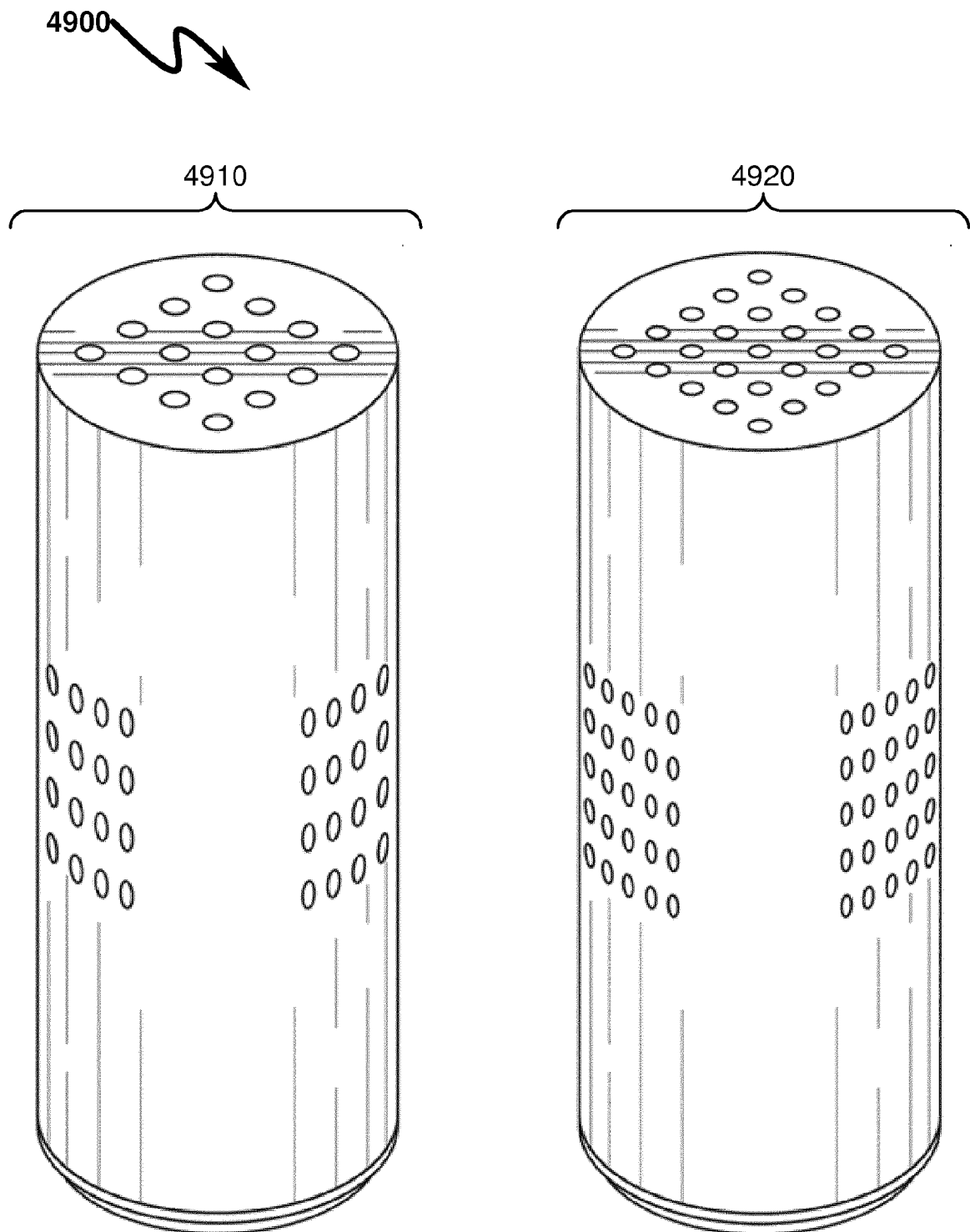
FIG. 49
