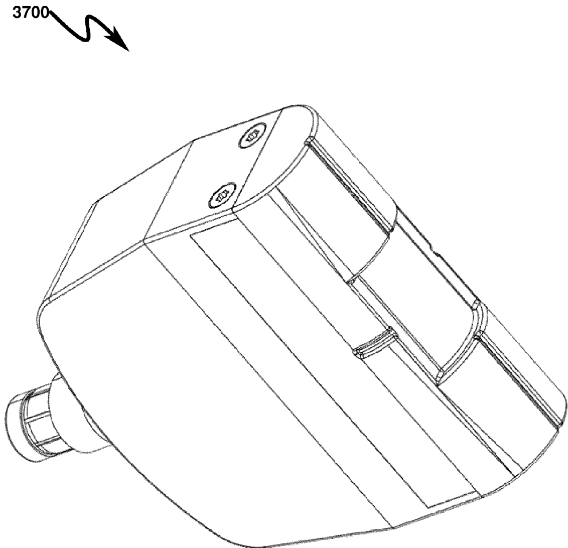
FIG. 37
